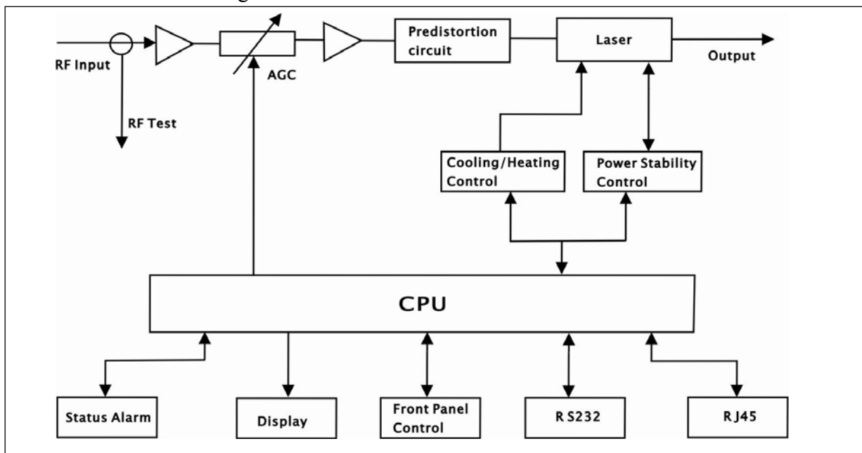
Bloc Diagram
