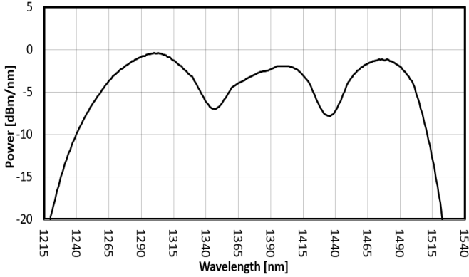
FIG. 1: ISB2 SPECTRUM
